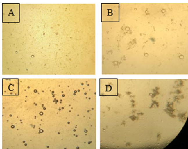
Fig. 2. Wall thickness of MCs with variation of CS:LGO:STPP (g); (A) 1:1:0.5, (B) 1:2:0.5, (C) 2:1:0.5, (D) 1:1:1
