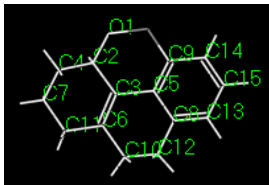
Fig. 1. ORTEP diagram
