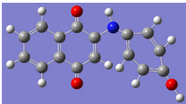
Fig. 2. 2-(4-Anilino)-1,4-naphthaquinone (ANQ)
