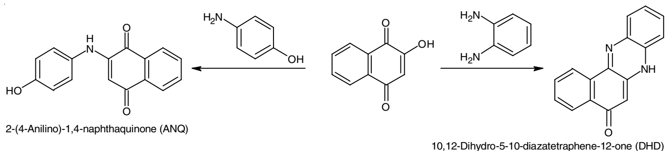
Scheme-I
